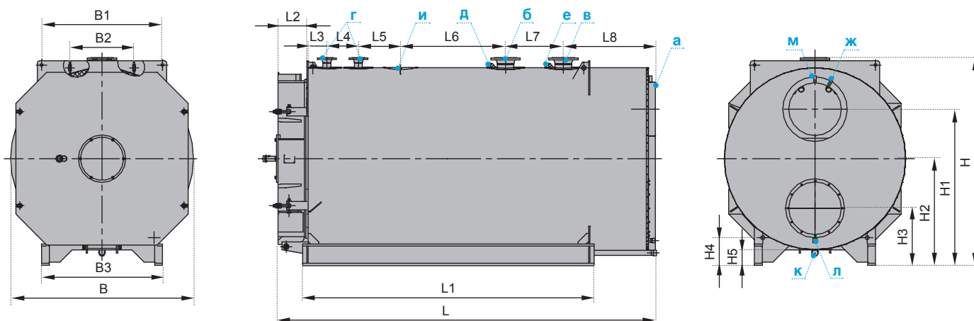
Рис. 3-а. Габаритные и присоединительные размеры
